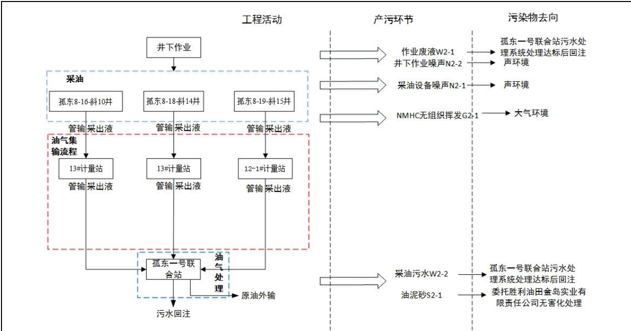
图 3-3 运营期主要工艺流程及产排污节点图
