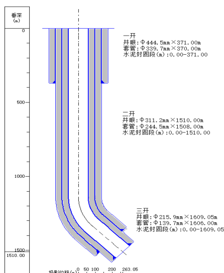
图 3-1 井身结构示意图
